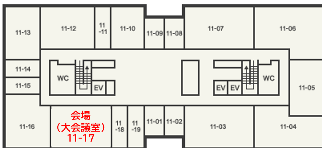
情報科学研究院棟（高層棟）11 階平面図
